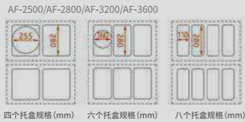
四个托盒规格(mm)
